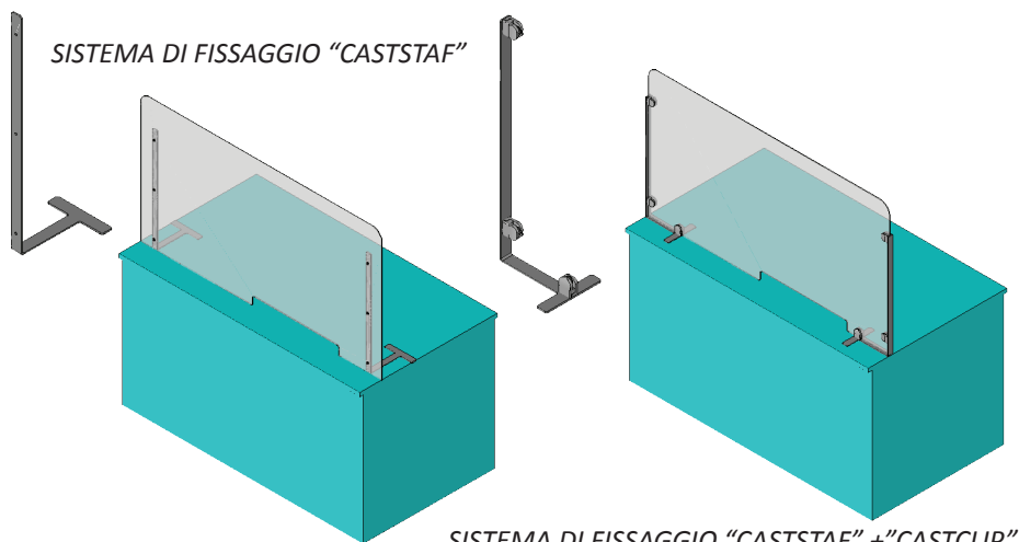
SISTEMA DI FISSAGGIO "CASTSTAF" + "CASTCLIP"
